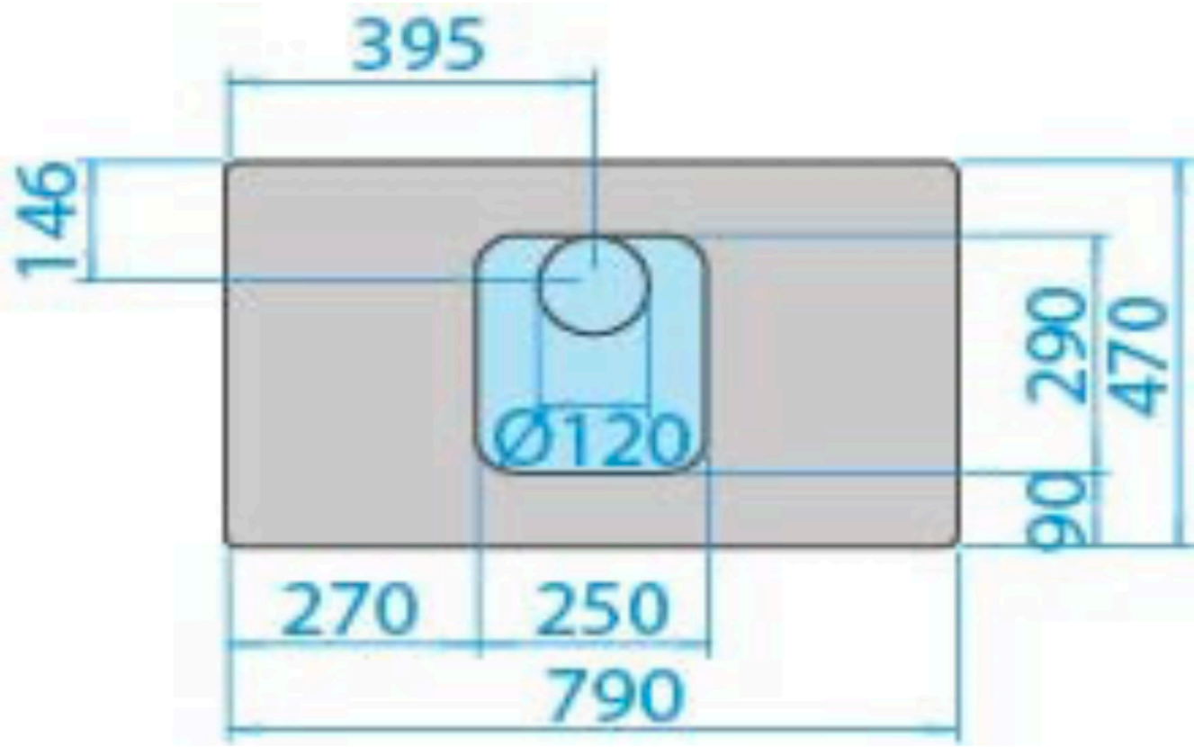
Maße Verbrennungsluft- Eintritt
