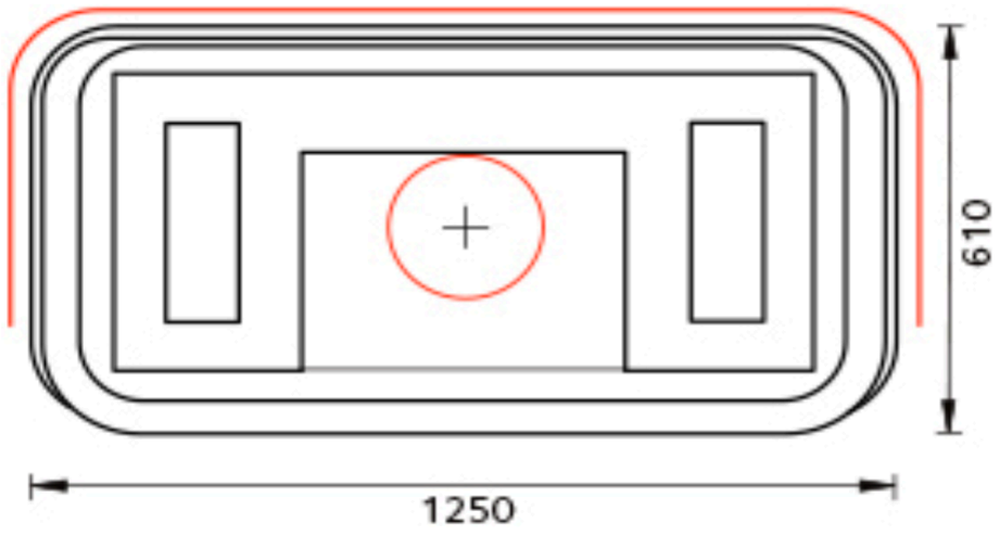
Grundriss (Anschlussbereich rot markiert)
