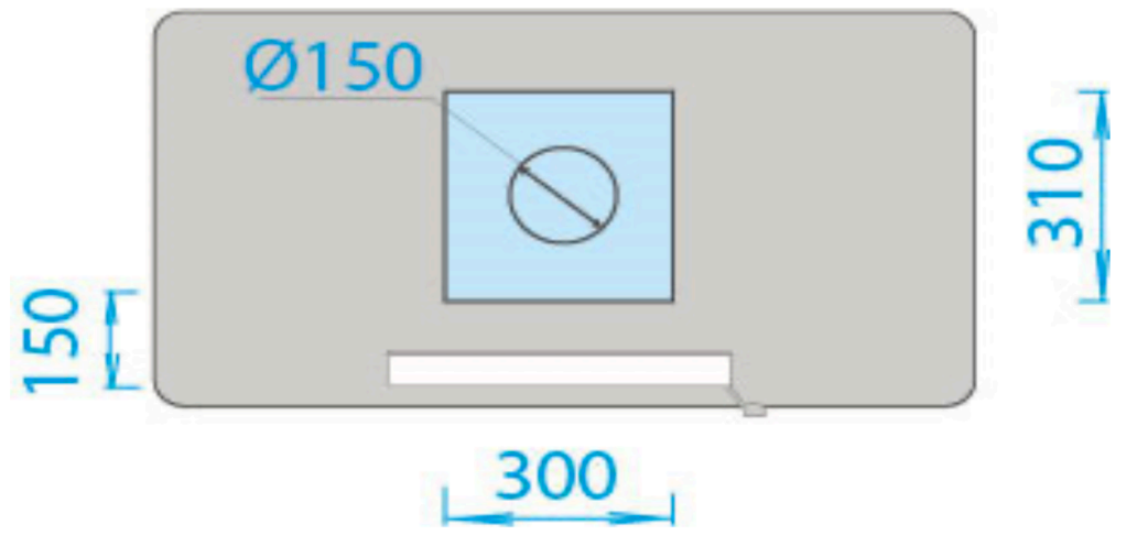
Maße Verbrennungsluft- Eintritt
