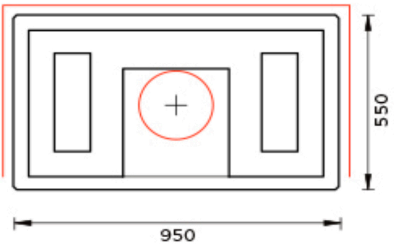
Grundriss (Anschlussbereich rot markiert)
