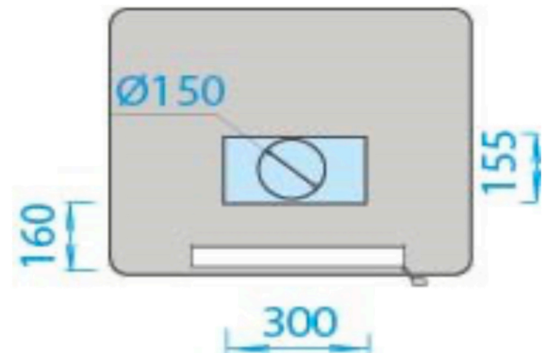
Maße Verbrennungsluft- Eintritt
