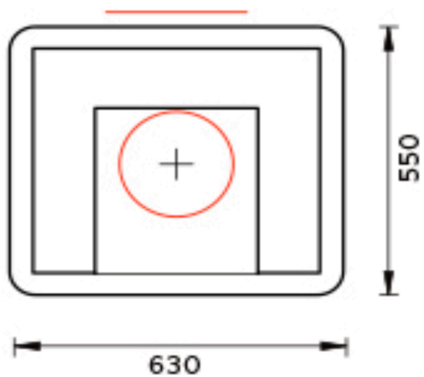
Grundriss (Anschlussbereich rot markiert)
