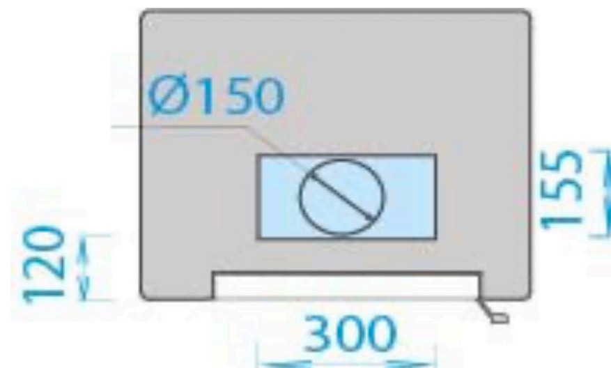
Maße Verbrennungsluft- Eintritt
